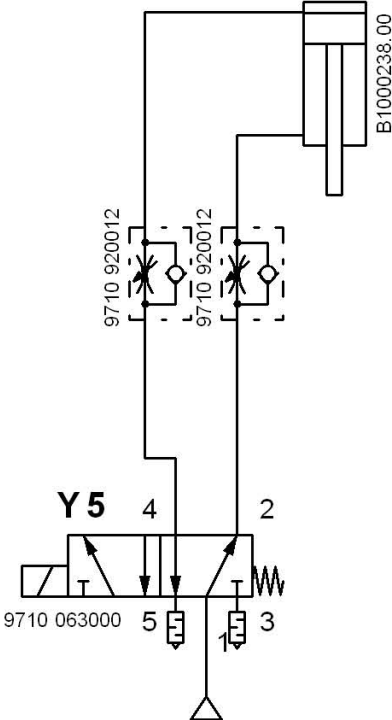
Fadenabschneider Unterfaden
