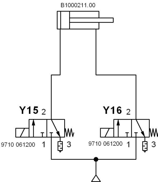
Nadelschaltung links rechts
